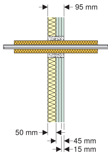
Billede 2: Dimensionering skaktvægge
