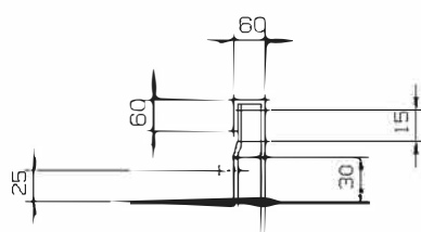
JOGGLE STRIP
